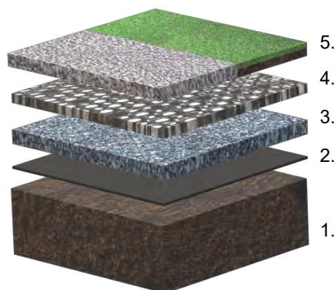
1. undergrund, 2. geotextil N2, 3. dränlager, 4. gräs- och grusarmering, 5. gräs/grus
