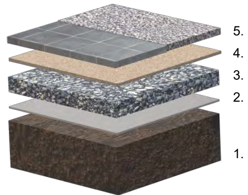
1. undergrund, 2. Typar® SF 3. förstärkningslager 4. justeringslager 5. marksten / sten
