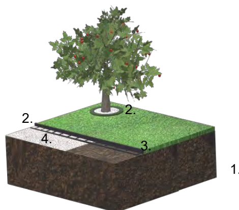
1. undergrund, 2. kantlist, 3. spik/fäste, 4. dekormaterial
