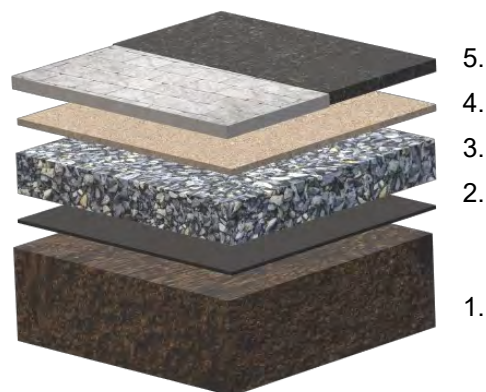
1. undergrund, 2. geotextil N2 3. förstärkningslager 4. justeringslager 5. marksten/asfalt
