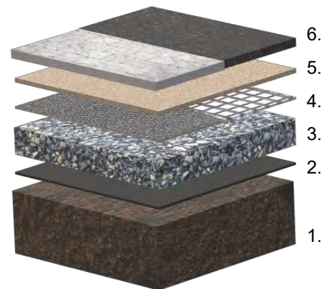
1. undergrund, 2. N2, 3. förstärkningslager, 4. markstensduk/geonät, 5. justeringslager, 6. marksten/asfalt
