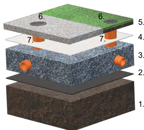
1. undergrund, 2. geotextil N2, 3. dräneringslager, 4. geotextil N1, 5. marklager 6. MIA betäckning, 7. dränrör/brunn
