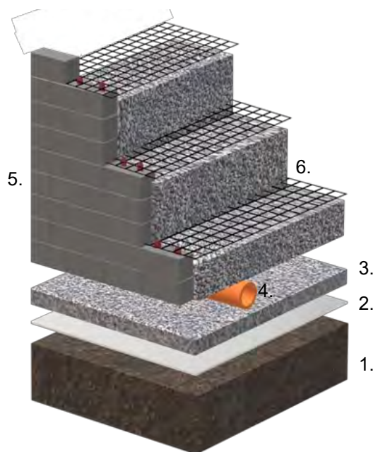
1. undergrund, 2. geotextil N2 3. makadam 4. dränrör 5. mur 6. geonät
