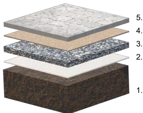
1. undergrund, 2. geotextil N1 3. förstärkningslager 4. justeringslager 5. marksten
